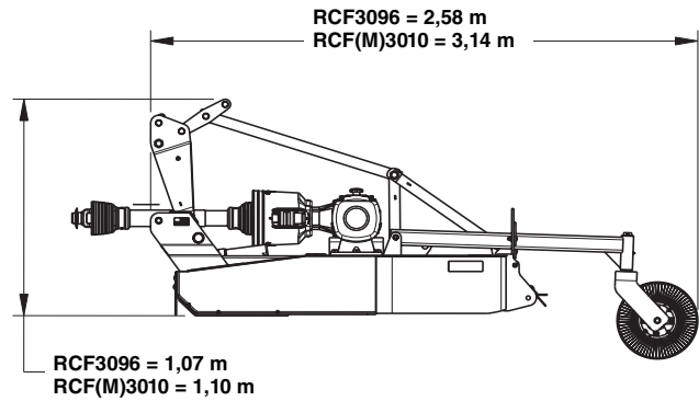
Débroussailleuse rotative à trois points (modèle RC3096 illustré)
