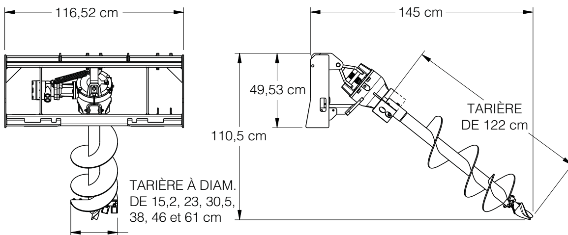
Bêche tarière montée sur chargeur à direction différentielle/tracto-chargeur, support central et décalé
