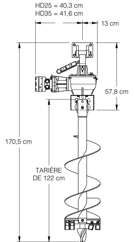
Bêche tarière à support de godet
