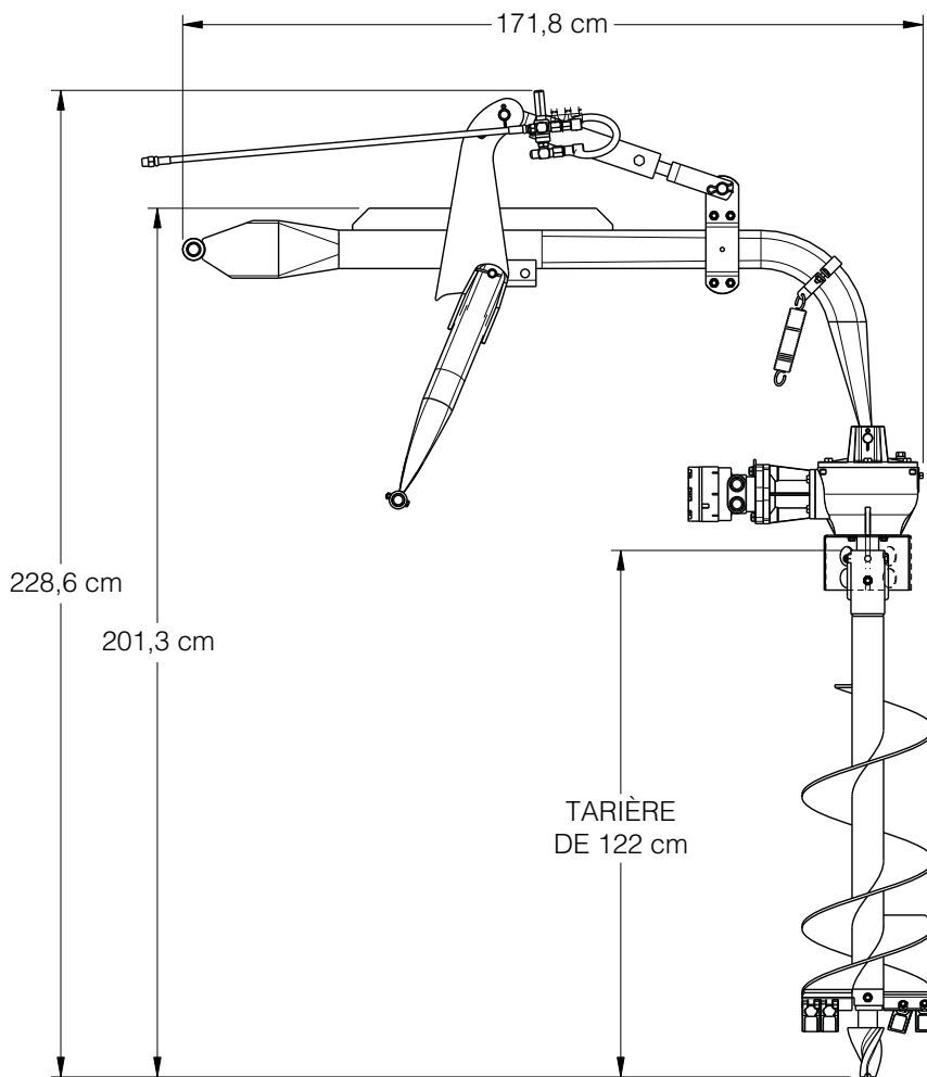
Bêche tarière à support à trois points
