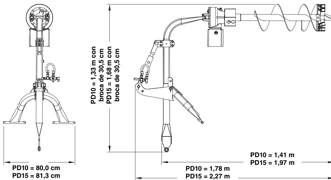
Dibujo dimensional general de las PD10 y PD15
