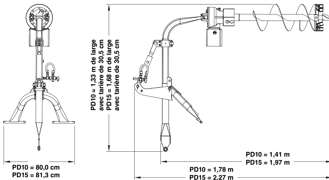
Dessin montrant les dimensions hors-tout PD10 et PD15
