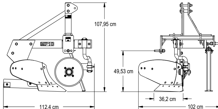
MP10 ARADO DE UNA SOLA VERTEDERA
