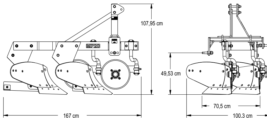
MP20 ARADO DE DOS VERTEDERAS
